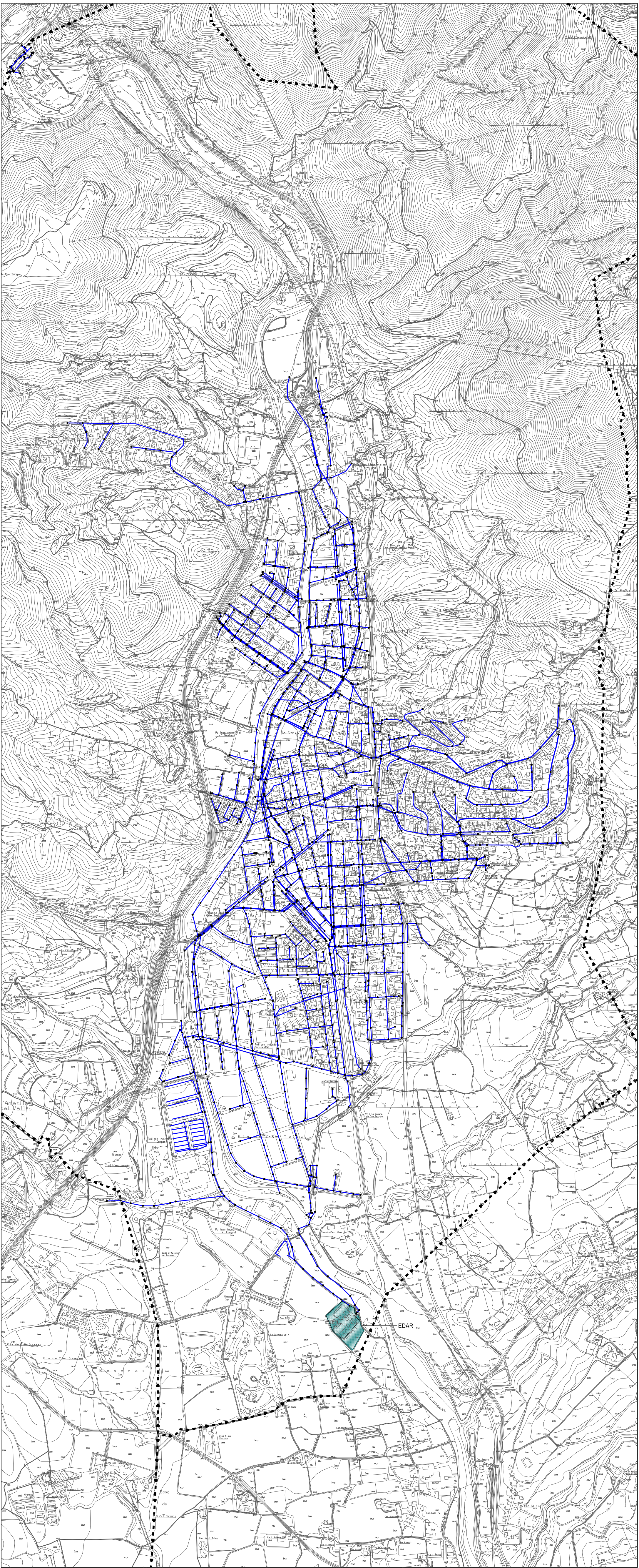
XARXA DE CLAVEGUERAM
